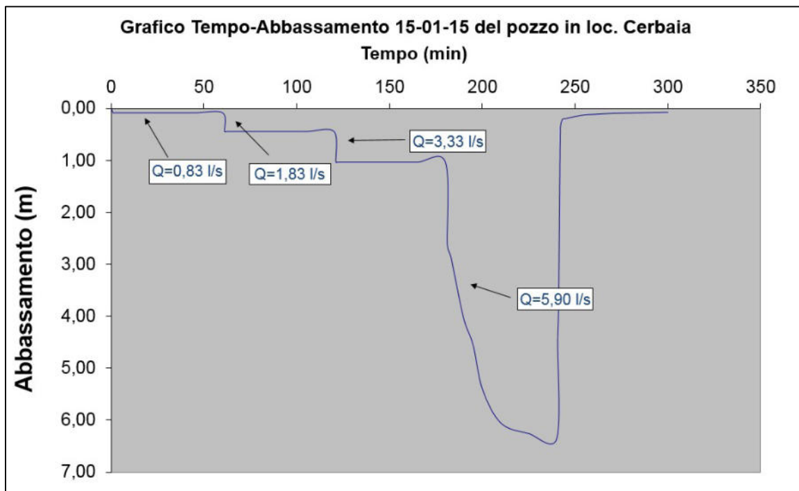
Fig. 15 – Grafico tempo abbassamento relativo alla prova di portata a gradini realizzata al pozzo PO595 del campo pozzi di Cerbaia
