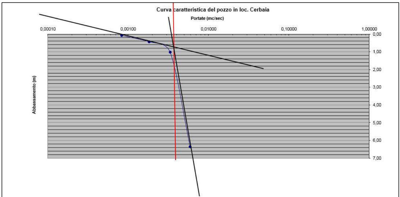
Fig. 17 - Curva caratteristica del pozzo PO595 in loc. Cerbaia
