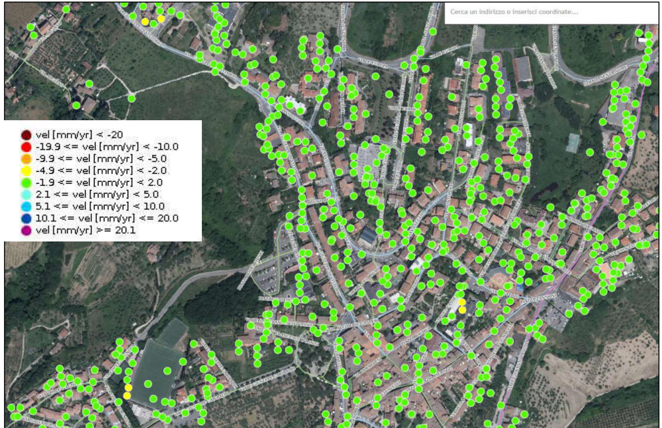
Fig. 8 - Prodotti interferometrici ENVISAT descending – Zona San Casciano in Val di Pesa (velocità media in mm/anno)
