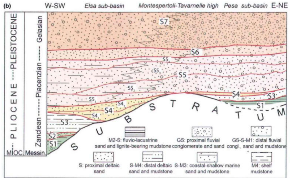
Fig. 2 – Schema stratigrafico della successione alto Messiniano – basso Pleistocene del bacino della Valdelsa mostrando l’architettura a sistemi dei sottobacini separati dall’alto Montespertoli-Tavarnelle (Benvenuti M. et al., 2014).
