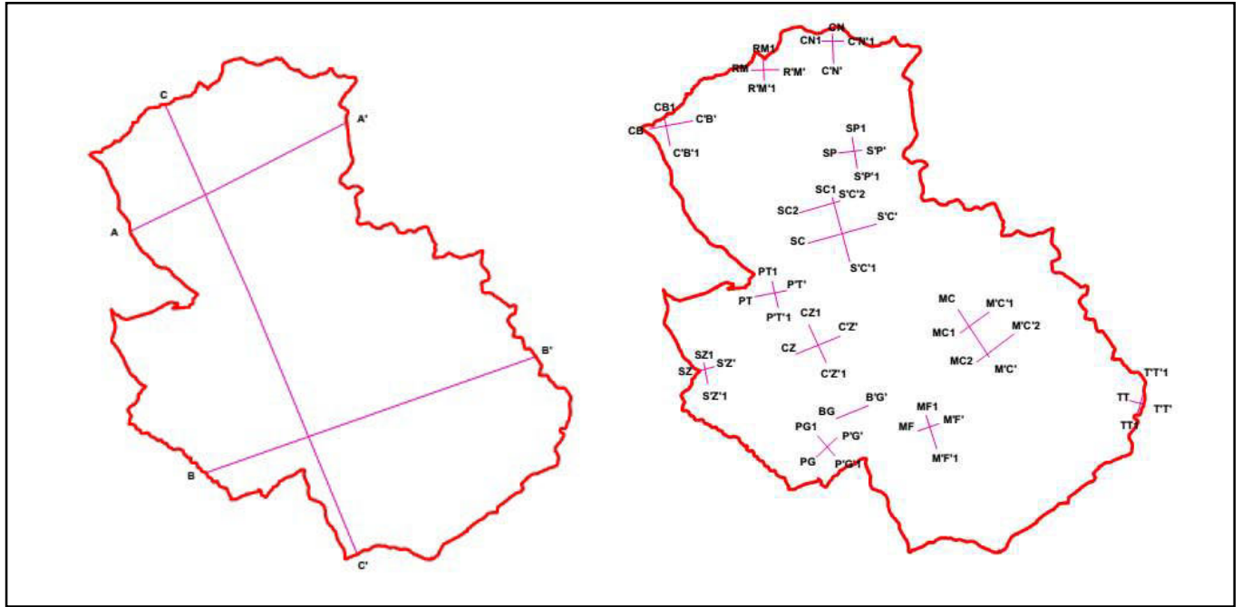
Fig. 21 – Ubicazione delle sezioni geologico-tecniche rappresentative
