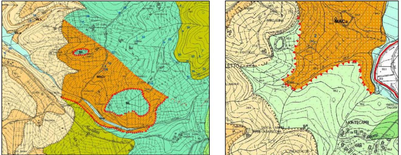
Fig. 4 – Sovrascorrimenti del Dominio Ligure sul Dominio Toscano nella porzione meridionale (a sinistra) e nella porzione orientale (a destra) del territorio comunale di San Casciano in Val di Pesa.
