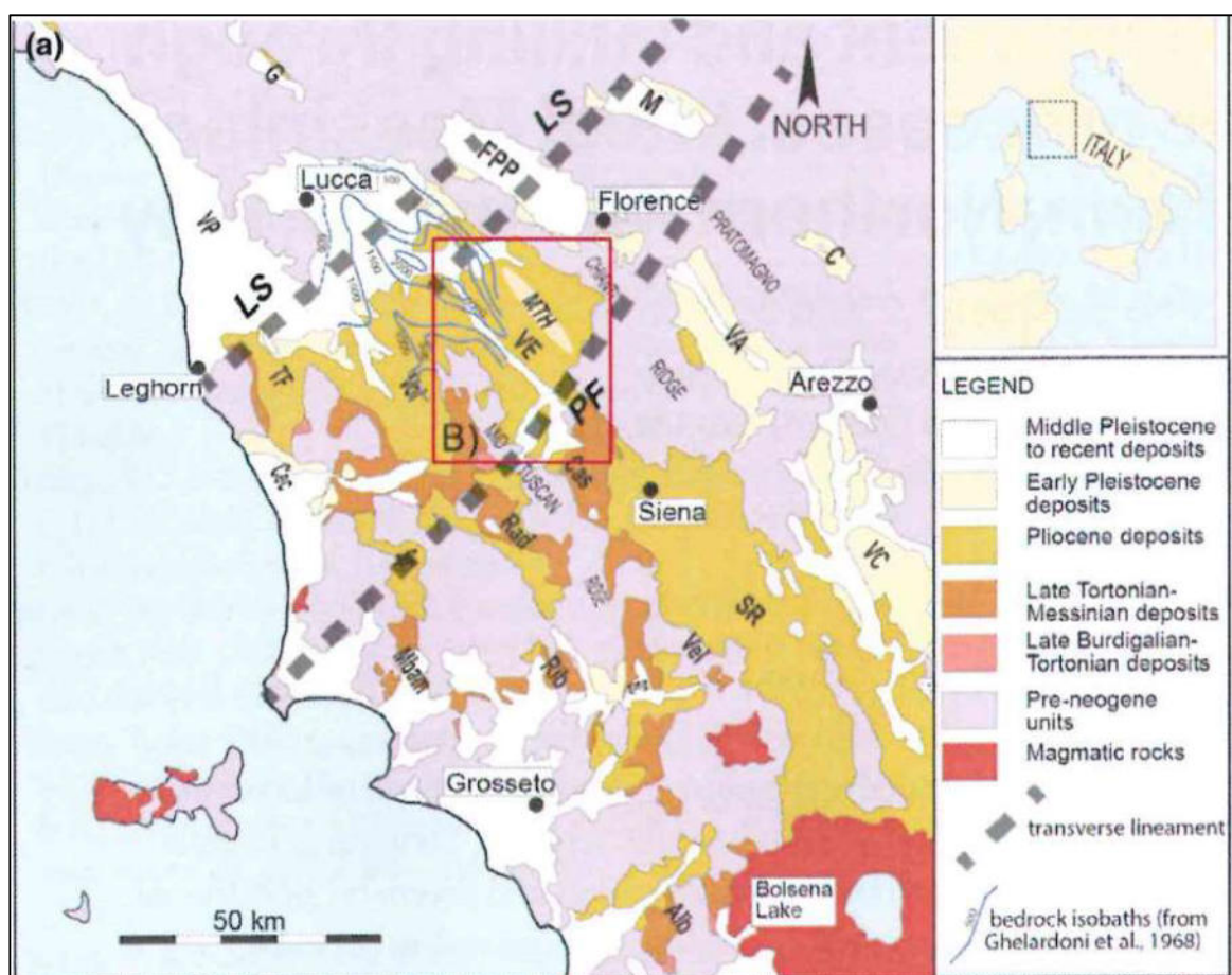
Fig. 1 – Distribuzione dei bacini Neogenici-quadernari della Toscana (Benvenuti M. et al., 2014).
