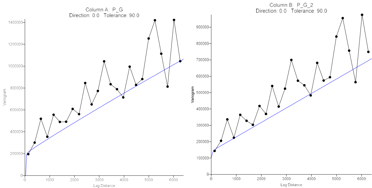
Fig. 24 – Semivariogrammi del potenziale geotermico. A destra semivariogramma per valori su 1800 h di estrazione. A sinistra semivariogramma con valori su 2400 h di estrazione.
