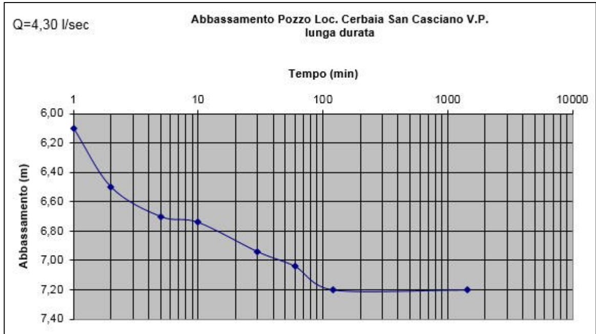
Fig. 16 - Grafico tempo abbassamento relativo alla prova a lunga durata a portata costante realizzata al pozzo PO595 del campo pozzi di Cerbaia
