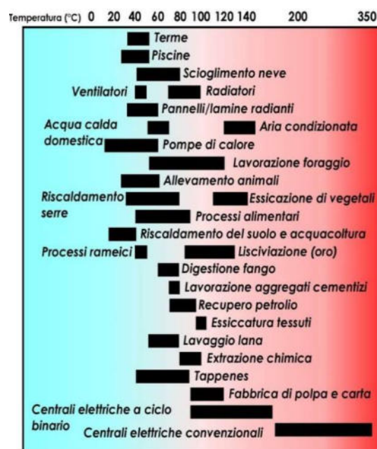
Fig. 22 – Applicazioni della risorsa geotermica in base all'entalpia del fluido reperito (Dickson M.H., 2004)
