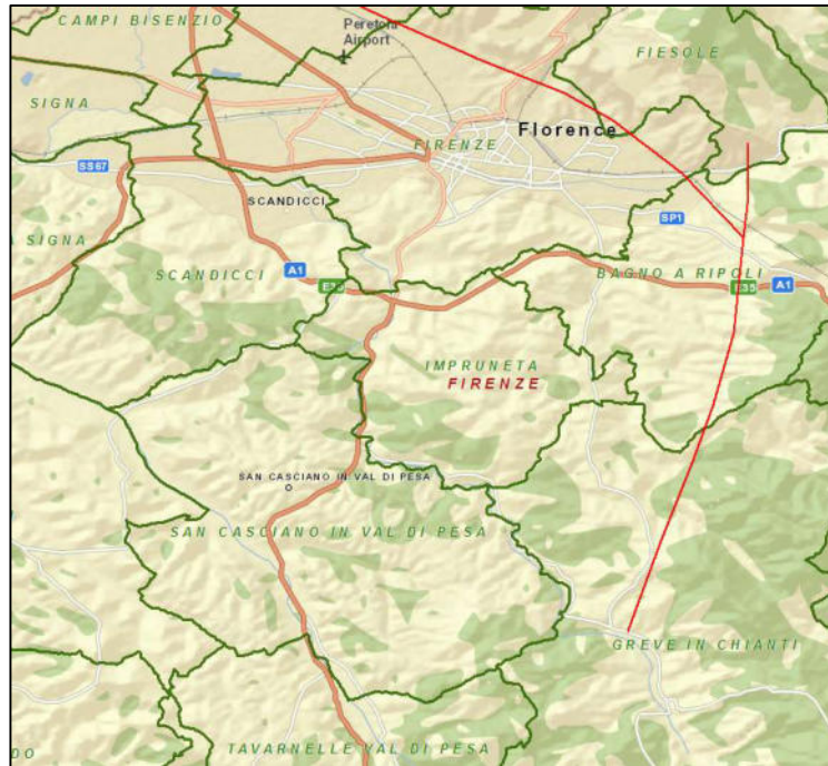
Fig. 20 – Estratto carta delle faglie attive capaci (in rosso) del Progetto ITHACA (fonte ISPRA).
