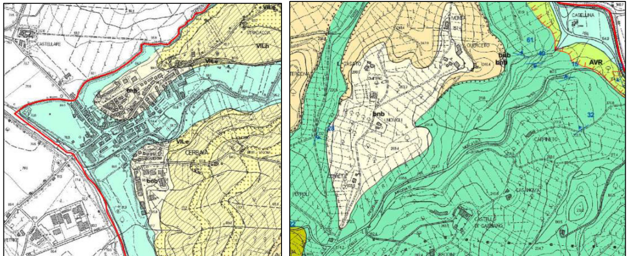
Fig. 3 – Affioramento dei depositi alluvionali recenti, terrazzati e non terrazzati (bnb) in loc. Cerbaia (a sinistra) e in loc. Novoli – Est di Mercatale in Val di Pesa (a destra)
